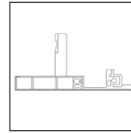
B591 لوازم اینتر ریل اسلیم شیشه با فرانت آلومینیوم و ارتفاع ۱۰۶mm سایز برش فرانت آلومینیومی : عرض داخل به داخل - ۹۷mm
