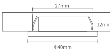
چراغ LED گرد نقطه ای سه تایی روکار و توکار همراه با ترانس مدل اورو (Oro) | N677 102,000,000R
