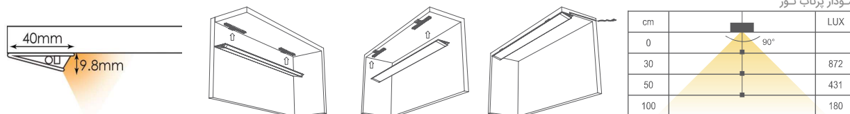
نمودار پرتاب نور
